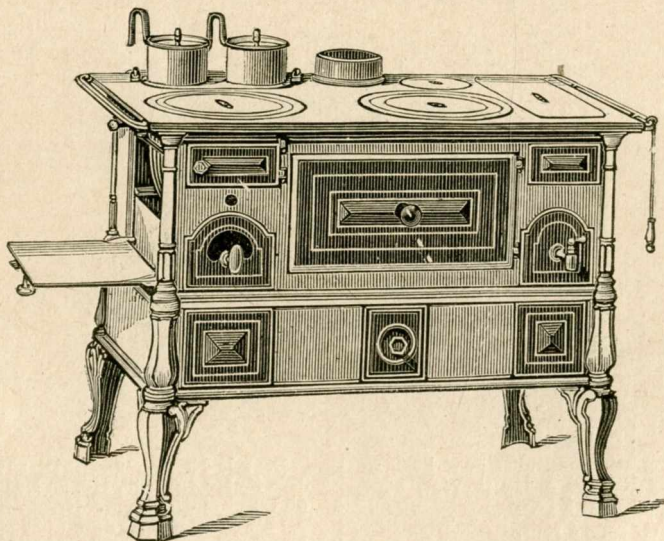
Les Cuisinières N os 114 et 116 ont le foyer à gauche
